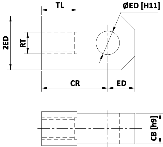
Piston Rod Eye (PRE)
